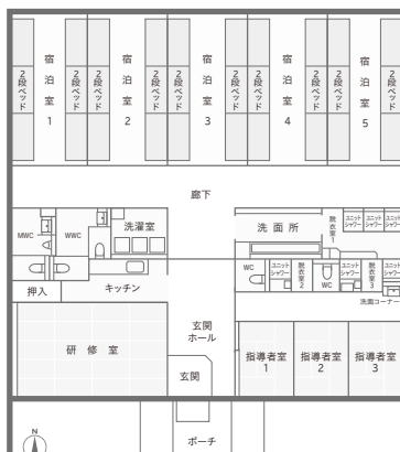
しらすぎセミナーハウス 平面図
